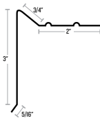
H6F DRIP EDGE
