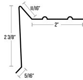
H5 1/2 DRIP EDGE
